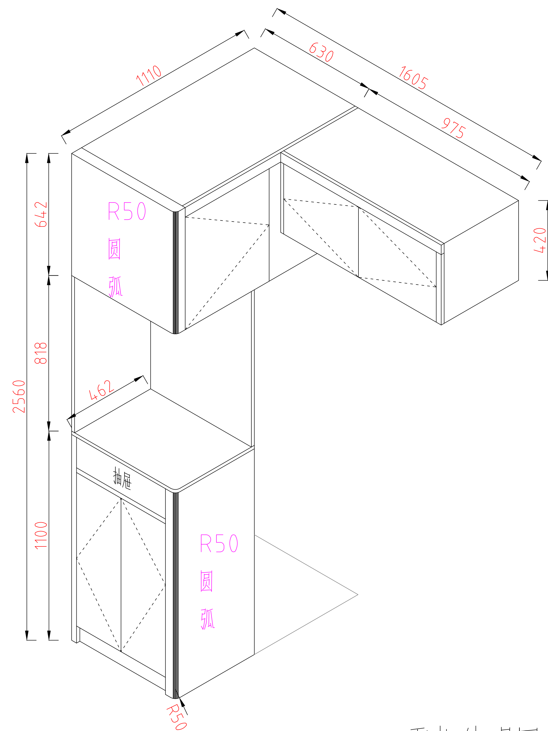
雪柜外观图
