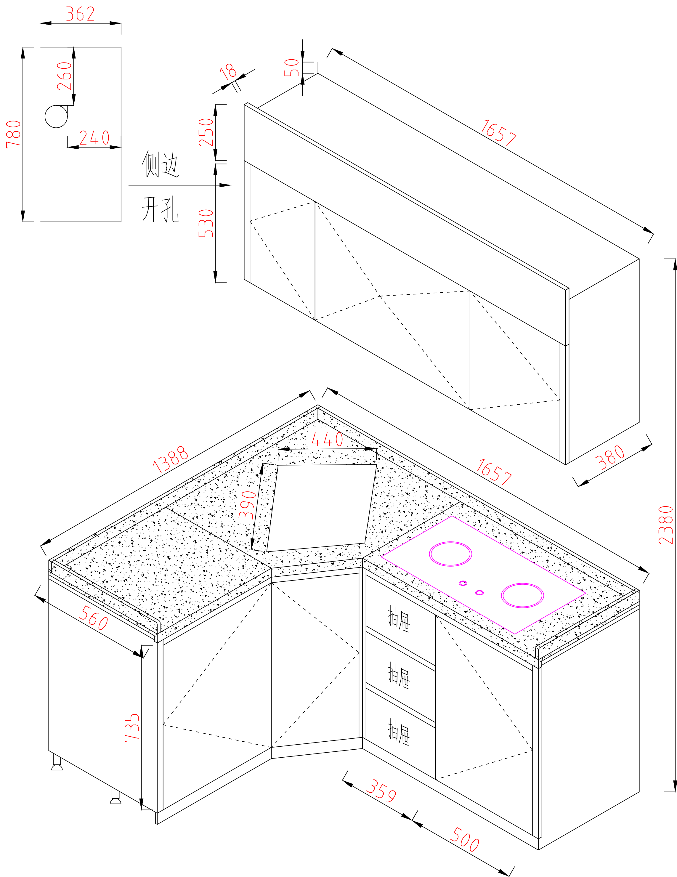
橱柜外观图
