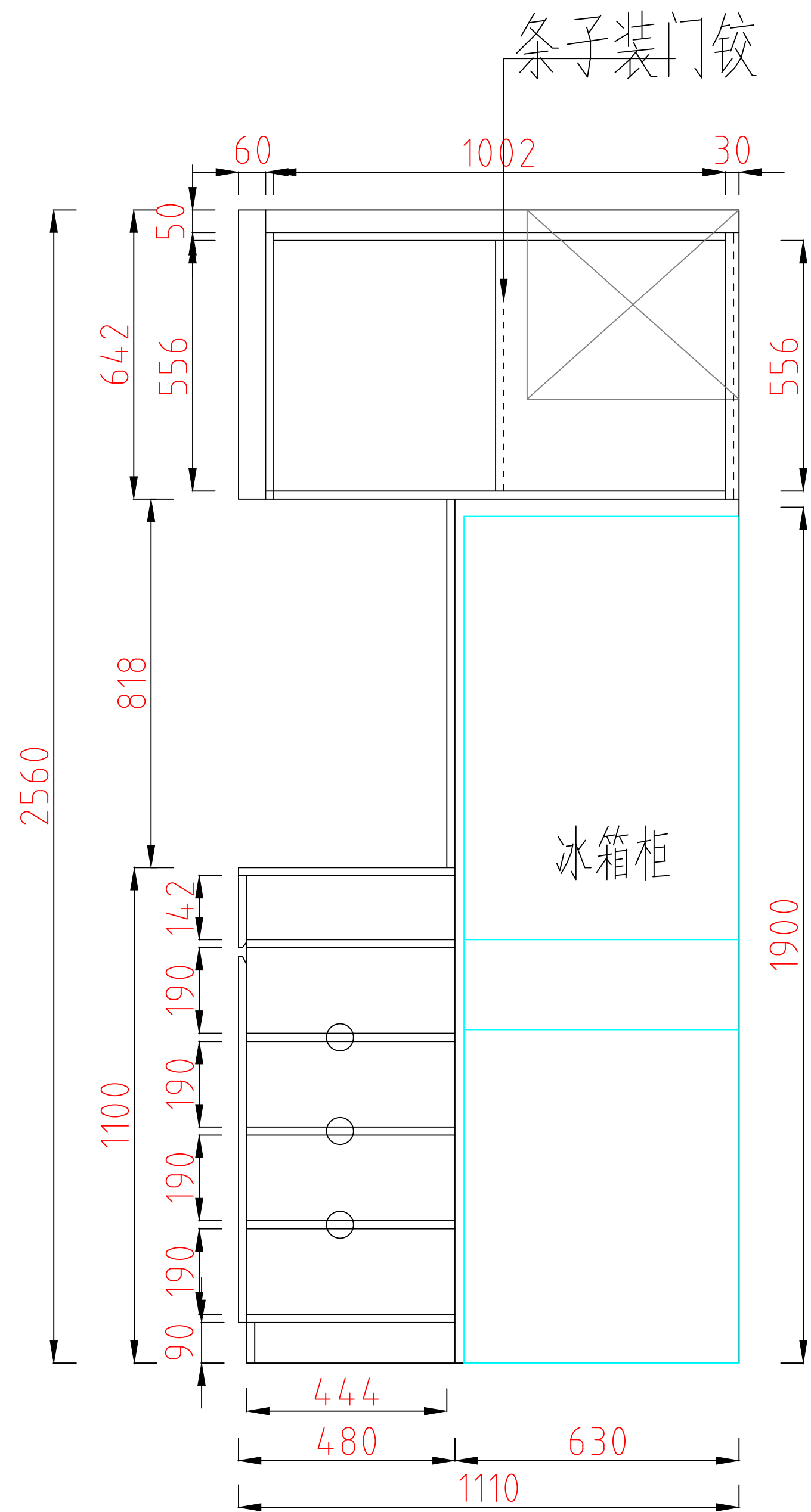
雪柜结构图
