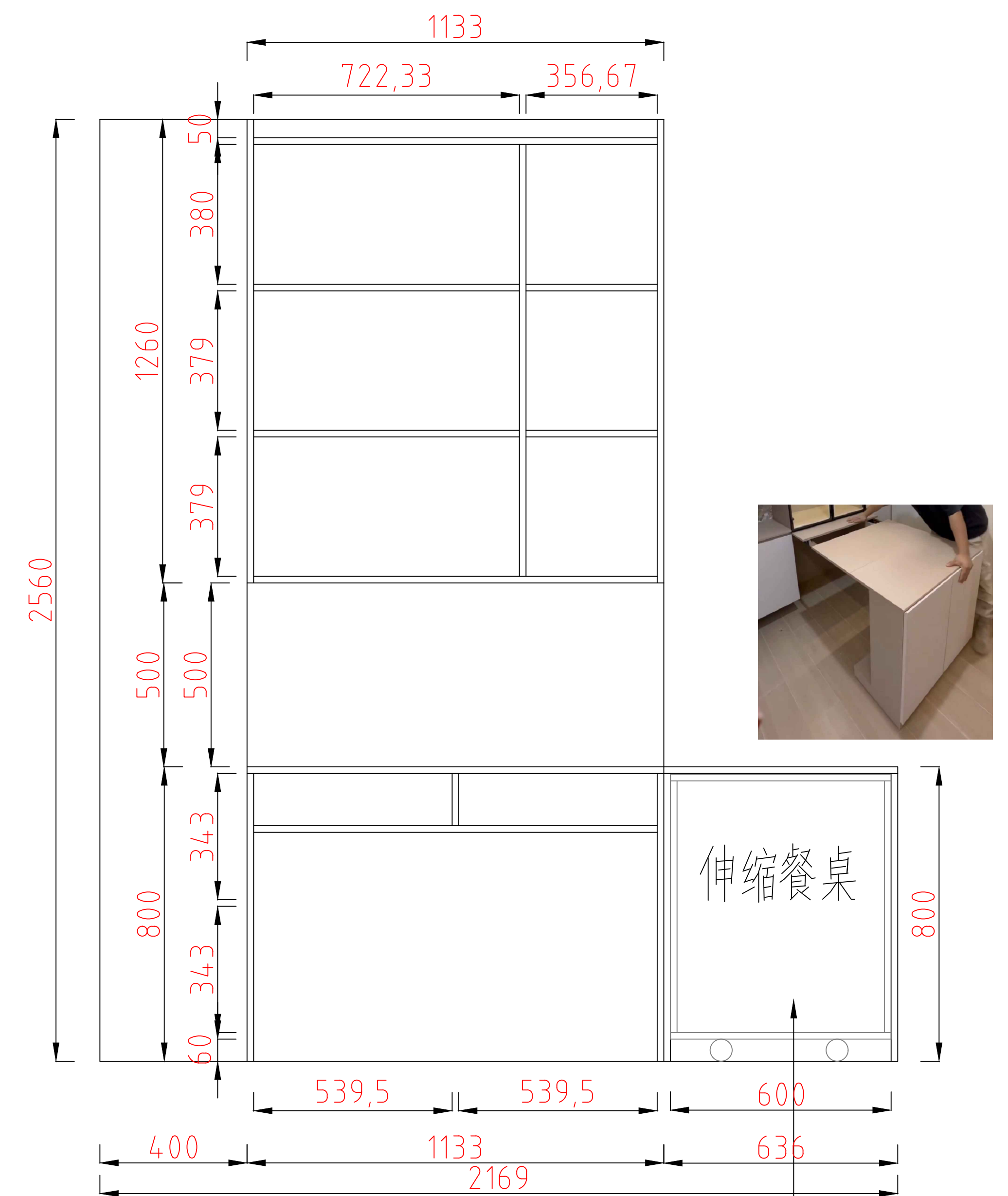
工作台加伸缩桌结构图
