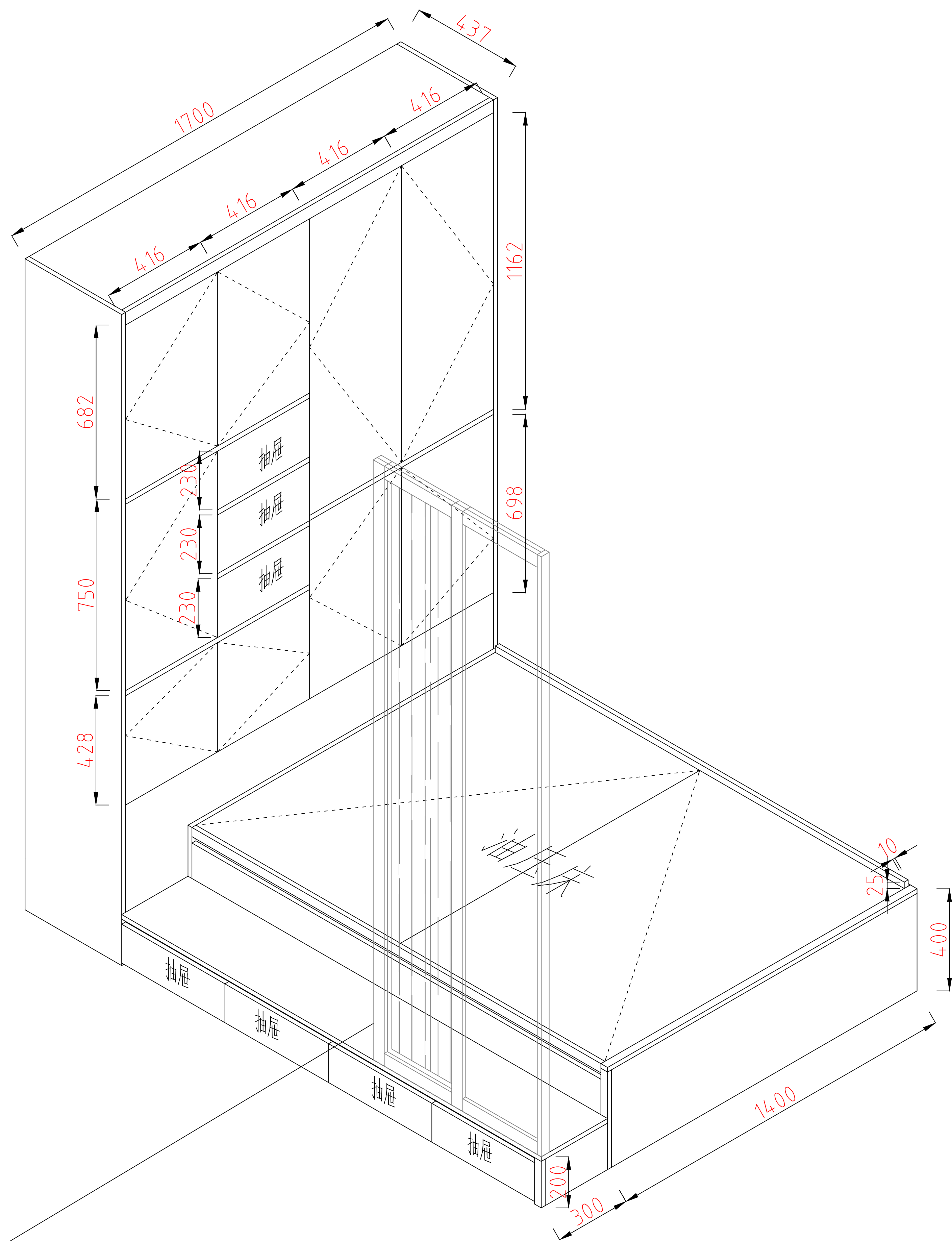
衣柜+油压床外观图
