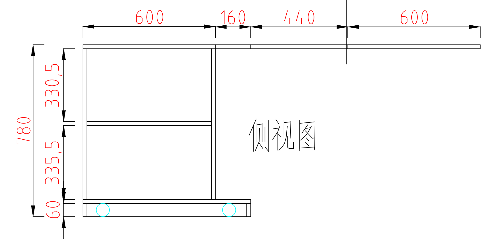
工作台加伸缩桌结构图
