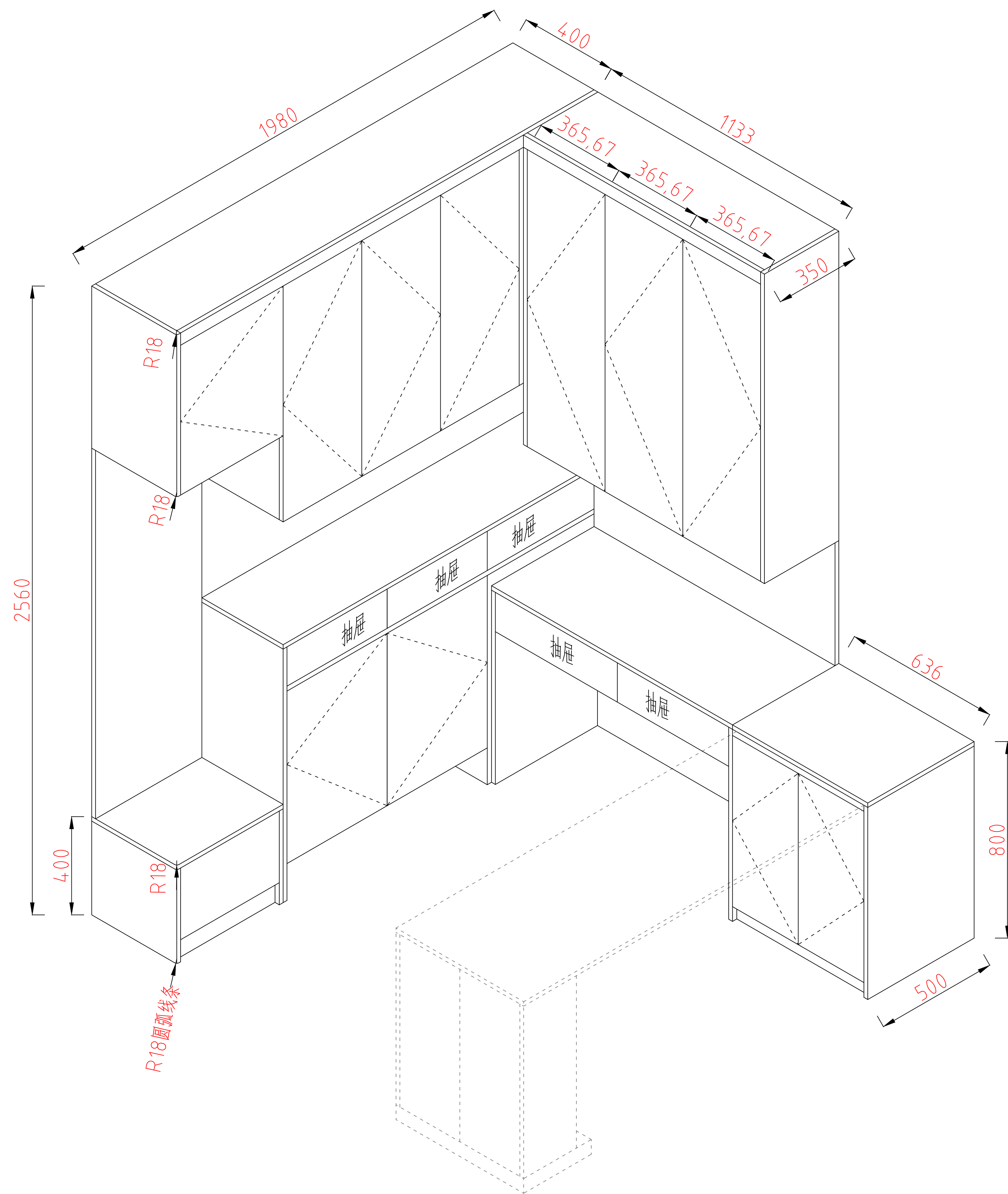
C字柜+工作台伸缩桌外观图
