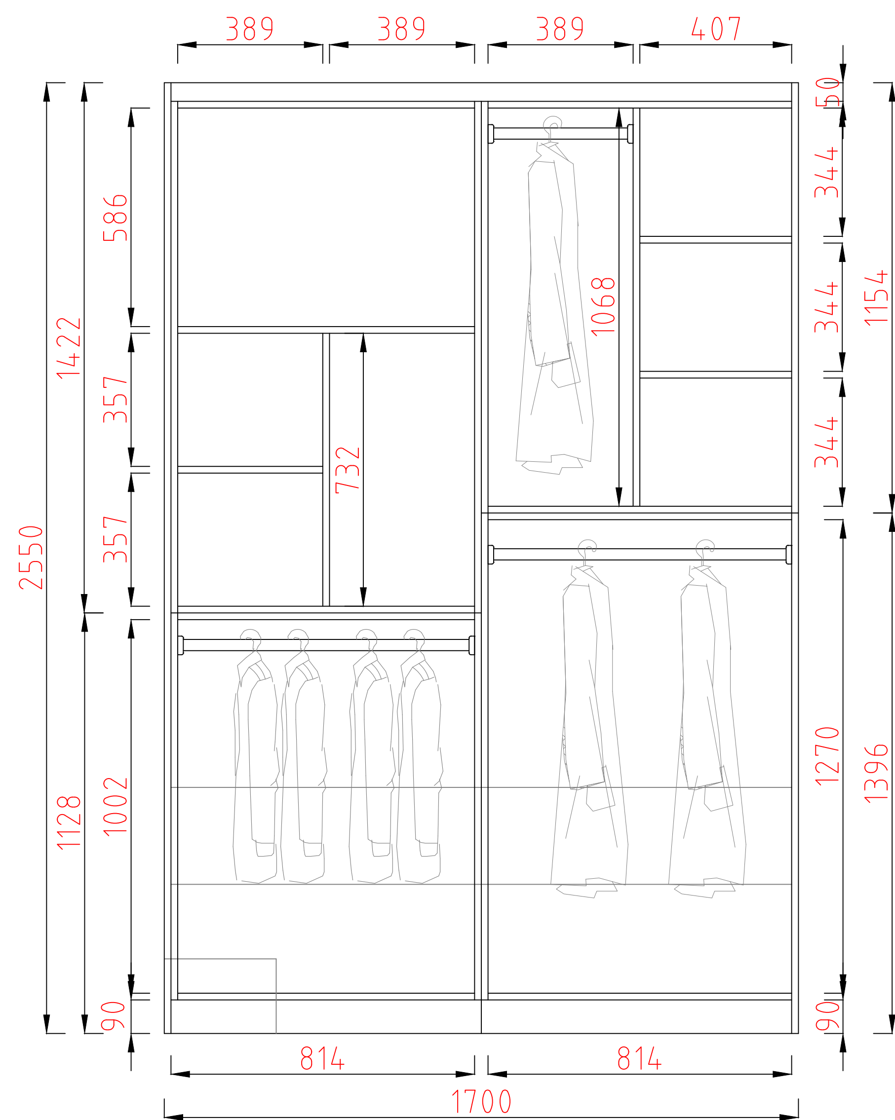
衣柜结构图
