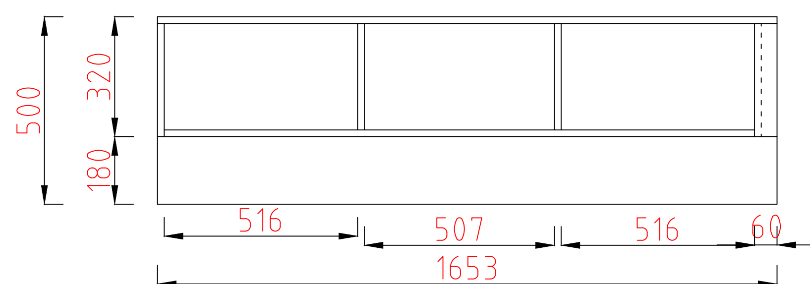
电视柜结构图
