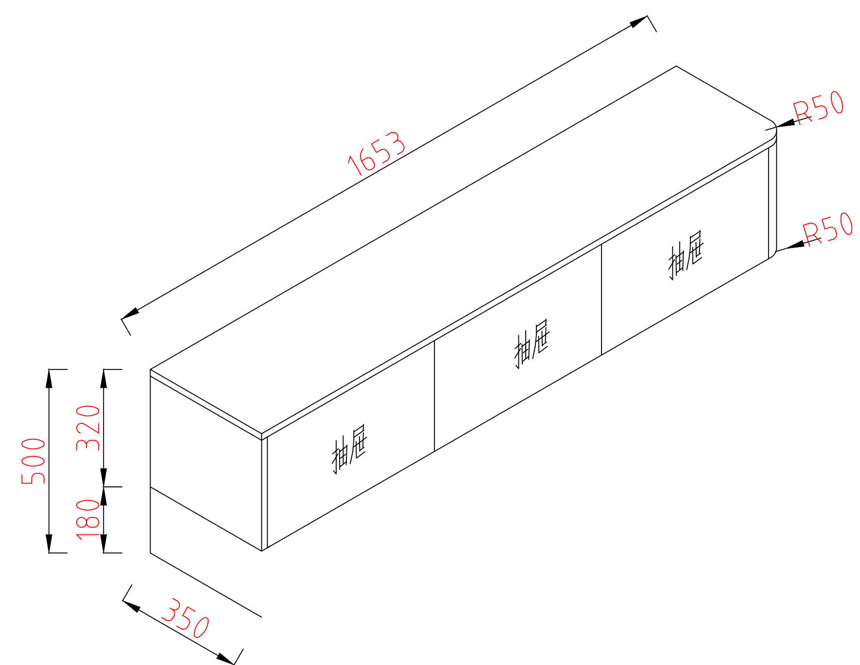
电视柜外观图
